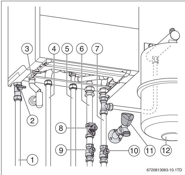
Rys. 1 Osprzęt przyłączeniowy (przykład)
